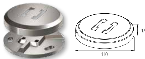
ΠΕΔΑΜΑ ΣΤΗΡΙΞΗΣ ΚΟΛΩΝΑΣ F50-108 SUPPORT FOOT FOR F50-108 COLUMN
