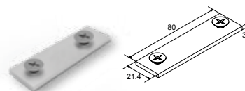
ΕΥΘΕΙΑ ΣΥΝΔΕΣΗΣ ΟΔΗΓΟΥ F50-319 LINEAR CONNECTOR FOR F50-319 GUIDE
