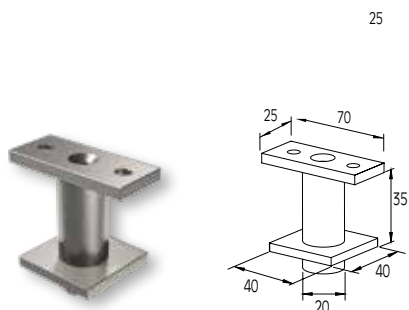
ΣΤΗΡΙΓΜΑ ΚΟΛΩΝΑΣ F50-102 ΜΕ ΚΟΥΠΑΣΤΗ F50-201 SUPPORT FOR F50-102 COLUMN WITH F50-201 HANDRAIL
