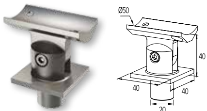
ΣΤΗΡΙΓΜΑ ΚΟΥΠΑΣΤΗΣ F50-200 ΜΕ ΚΟΛΩΝΑ F50-102 (ΣΚΑΛΑ) SUPPORT FOR F50-200 HANDRAIL WITH F50-102 COLUMN (STAIRS)
