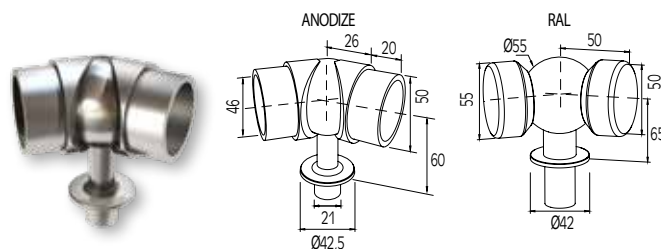
ΣΥΝΔΕΣΜΟΣ ΜΕΤΑΒΛΗΤΗΣ ΓΩΝΙΑΣ ΚΟΥΠΙΑΣΤΗΣ Ø50 ΜΕ ΚΟΛΩΝΑ Ø42 ADJUSTABLE CORNER CONNECTOR FOR HANDRAIL Ø50 WITH COLUMN Ø42
