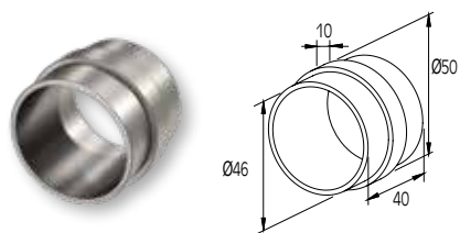
ΕΣΩΤΕΡΙΚΟΣ ΣΥΝΔΕΣΜΟΣ ΚΟΥΠΑΣΤΩΝ Ø50 CONNECTOR FOR HANDRAIL Ø50 (INTERNAL)
