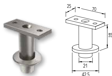
ΣΥΝΔΕΣΜΟΣ ΚΟΛΩΝΑΣ F50-100 ΜΕ ΚΟΥΓΙΑΣΤΗ F50-201 CONNECTOR FOR F50-100 COLUMN WITH F50-201 HANDRAIL
