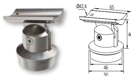
ΣΥΝΔΕΣΜΟΣ ΚΟΛΩΝΑΣ F50-100 ΜΕ ΚΟΥΓΙΑΣΤΗ F50-200 CONNECTOR FOR F50-100 COLUMN WITH F50-200 HANDRAIL
