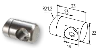
ΣΥΝΔΕΣΜΟΣ ΚΟΛΩΝΑΣ F50-100 ΜΕ ΠΡΟΦΙΛ Ø16 CONNECTOR FOR F50-100 COLUMN WITH PROFILE Ø16
