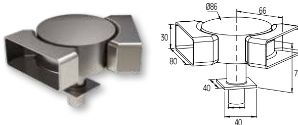
ΣΥΝΔΕΣΜΟΣ ΜΕΤΑΒΛΗΤΗΣ ΓΩΝΙΑΣ ΚΟΥΠΑΣΤΗΣ 80x30 ΜΕ ΚΟΛΩΝΑ F50-102 ADJUSTABLE CORNER CONNECTOR FOR 80x30 HANDRAIL WITH F50-102 COLUMN
