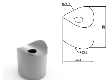
ΣΥΝΔΕΣΜΟΣ F50-307/327 ΜΕ ΚΟΛΩΝΑ F50-103/123 CONNECTOR FOR F50-307-327 WITH F50-103/123 COLUMN
