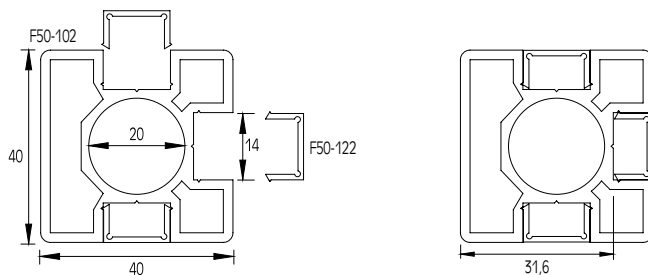
ΚΑΠΑΚΙ ΚΟΛΩΝΑΣ F50-102 COVER FOR F50-102 COLUMN
