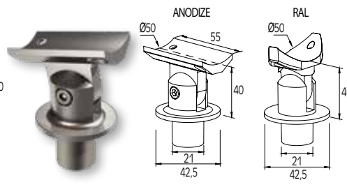
ΣΥΝΔΕΣΜΟΣ ΚΟΥΠΙΑΣΤΗΣ Ø50 ΜΕ ΚΟΛΩΝΑ Ø42 (ΣΚΑΛΑ) CONNECTOR FOR HANDRAIL Ø50 WITH COLUMN Ø42 (STAIRS)
