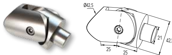
ΣΥΝΔΕΣΜΟΣ ΚΟΛΩΝΑΣ ΜΕ ΚΟΛΩΝΑ F50-100 (ΣΚΑΛΑ) CONNECTOR FOR COLUMN WITH COLUMN F50-100 (STAIRS)
