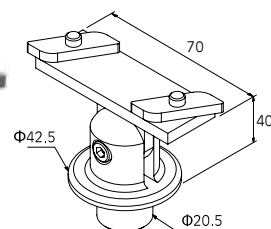
ΣΤΗΡΙΓΜΑ ΚΟΥΠΑΣΤΗΣ F50-201 ΜΕ ΚΟΛΩΝΑ F50-100 (ΣΚΑΛΑ) SUPPORT FOR F50-201 HANDRAIL WITH F50-100 COLUMN (STAIRS)
