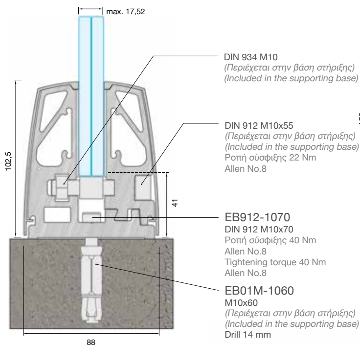
Διατομή υαλοπίνακα τύπου A Glass section A
