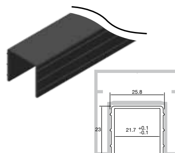
EPDM GASKET Κωδικός/Code F85-465
