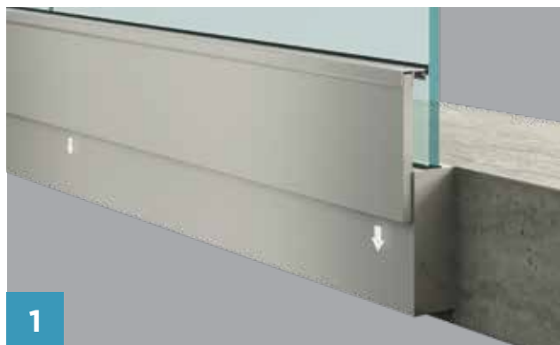
1 Τοποθέτηση του προφίλ επικάλυψης / Placing the top cover profile
