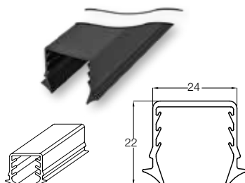
Λάστιχο "U" "U" shaped gasket Κωδικός/Code F85-407 (10.10.4)
