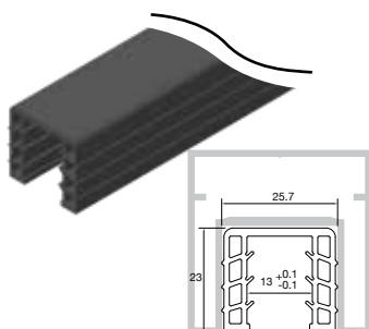
EPDM GASKET Κωδικός/Code F85-463
