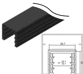
EPDM GASKET Κωδικός/Code F85-464
