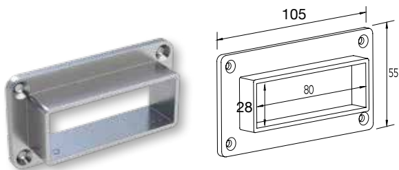
ΑΡΜΟΚΑΛΥΠΤΡΟ ΚΟΥΠΑΣΤΗΣ CLS-202 WALL COVER FOR CLS-202 HANDRAIL Κωδ. / Code 4533(Z)
