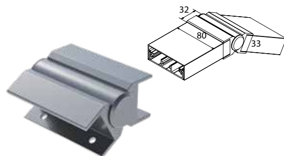
ΣΥΝΔΕΣΜΟΣ ΜΕΤΑΒΛΗΤΟΣ ΓΙΑ ΚΟΥΠΙΑΣΤΗ CLS-202 ADJUSTABLE CONNECTOR FOR HANDRAIL CLS-202
