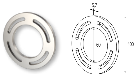
ΡΟΖΕΤΑ ΤΖΑΜΙΟΥ Ø100 GLASS ROSETTE Ø100 Κωδ. / Code 4611
