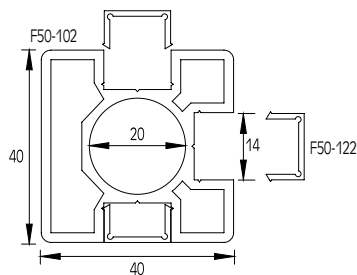
ΚΑΠΑΚΙ ΚΟΛΩΝΑΣ F50-102 COVER FOR F50-102 COLUMN
