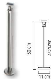
ΕΤΟΙΜΗ ΚΟΛΩΝΑ ΓΙΑ Ø16 ΠΡΟΦΙΛ ΥΨΟΣ 50 cm READY MADE COLUMN FOR Ø16 PROFILE HEIGHT 50 cm Κωδ. / Code 4620-050
