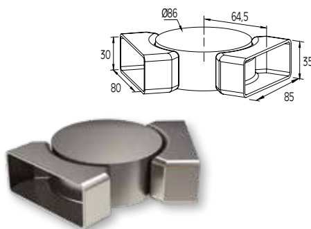
ΣΥΝΔΕΣΜΟΣ ΜΕΤΑΒΛΗΤΗΣ ΓΩΝΙΑΣ ΚΟΥΠΑΣΤΗΣ F50-203 ADJUSTABLE CORNER CONNECTOR FOR F50-203 HANDRAIL
