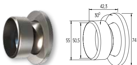
ΑΡΜΟΚΑΛΥΠΤΡΟ ΚΟΥΠΑΣΤΗΣ Ø50 (ΜΕ ΚΑΠΑΚΙ) WALL COVER FOR HANDRAIL Ø50 WITH CAP Κωδ. / Code 4518
