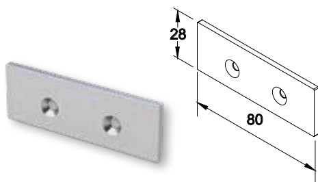
Τάπα κουπαστής CLS-202 End cap for F50-201 handrail
