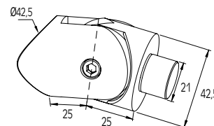
ΣΥΝΔΕΣΜΟΣ ΚΟΛΩΝΑΣ ΜΕ ΚΟΛΩΝΑ F50-100 (ΣΚΑΛΑ) CONNECTOR FOR COLUMN WITH COLUMN F50-100 (STAIRS)
