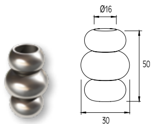
ΡΟΖΕΤΑ ΓΙΑ ΠΡΟΦΙΛ Ø16 ROSETTE FOR PROFILE Ø16 Κωδ. / Code 4618
