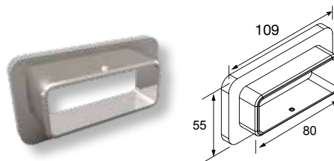
ΑΡΜΟΚΑΛΥΠΤΡΟ ΚΟΥΠΑΣΤΗΣ F50-201/203 (ΜΕ ΚΑΠΑΚΙ) WALL COVER FOR F50-201/203 HANDRAIL (WITH CAP) Κωδ. / Code 4515Z
