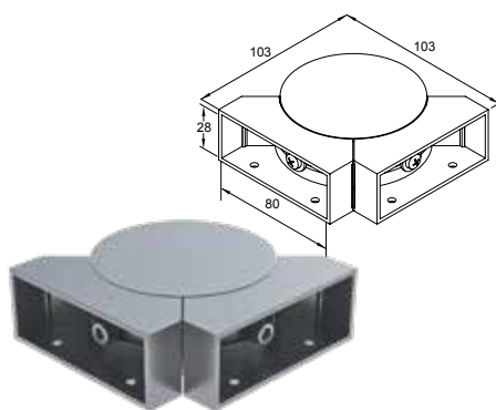
ΣΥΝΔΕΣΜΟΣ ΜΕΤΑΒΛΗΤΗΣ ΓΩΝΙΑΣ ΚΟΥΠΑΣΤΩΝ CLS-202 ADJUSTABLE CORNER CONNECTOR FOR HANDRAIL CLS-202
