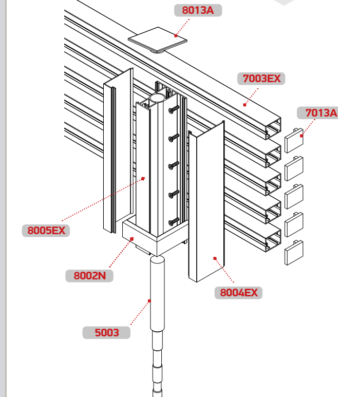
Συνδεσμολογία κολώνας SD-8005EX με SD-7003EX προφίλ. Column SD-8005EX Assembling with SD-7003EX profile
