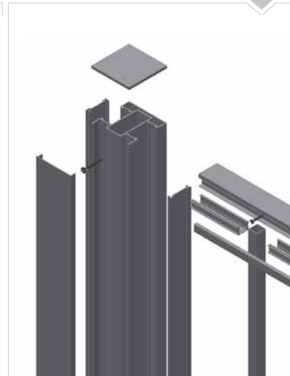
Συνδεσμολογία κολώνας SD-9005N με SD-403M προφίλ. Column SD-9005N Assembling with SD-403M profile
