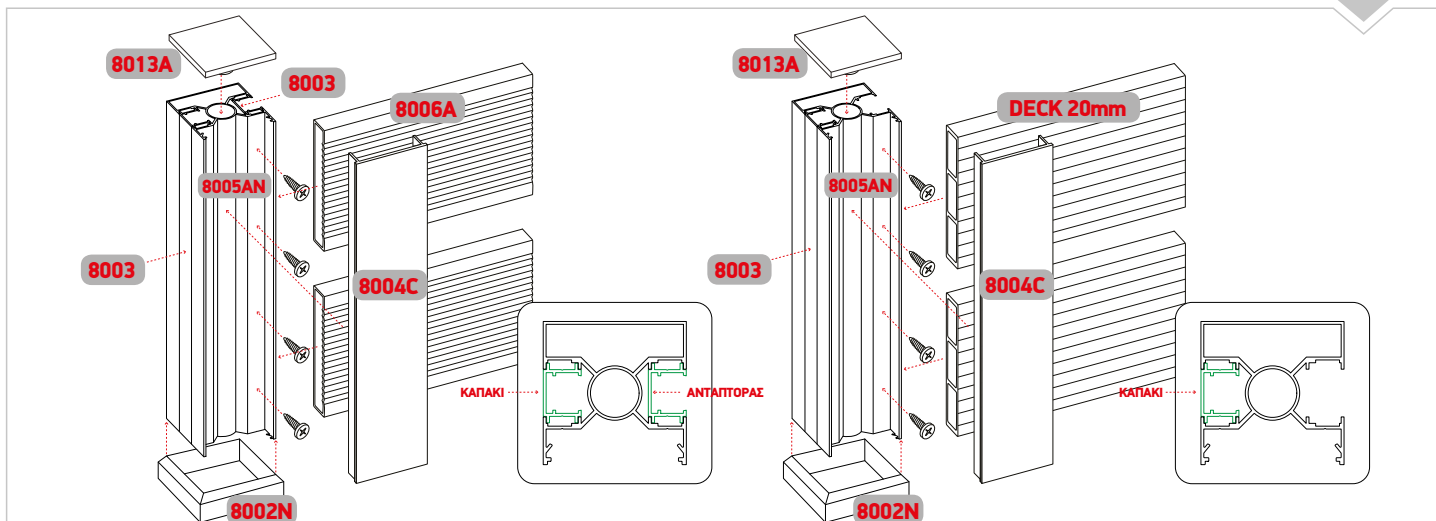
Συνδεσμολογία κολώνας SD-8005AN με SD-8006A προφίλ. Column SD-8005AN Assembling with SD-8006A profile
