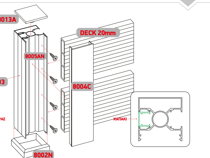
Συνδεσμολογία κολώνας SD-8005AN με SD-8006N προφίλ. Column SD-8005AN Assembling with SD-8006N profile
