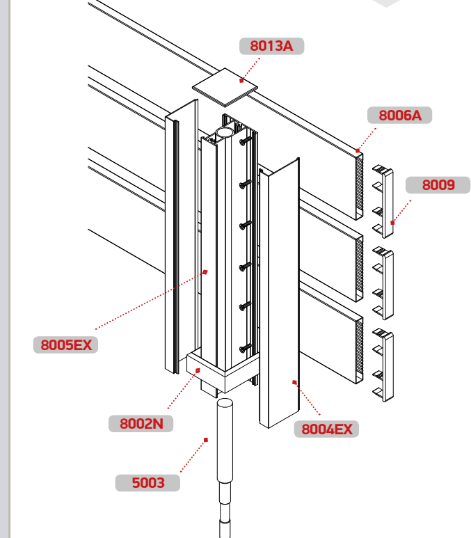
Συνδεσμολογία κολώνας SD-8005EX με SD-8006A προφίλ. Column SD-8005EX Assembling with SD-8006A profile
