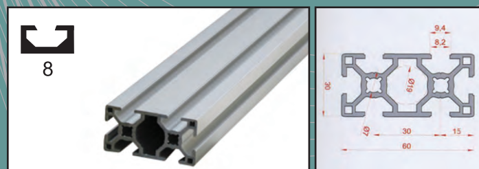
30X60 profile
