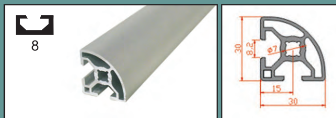
30X30 radius
