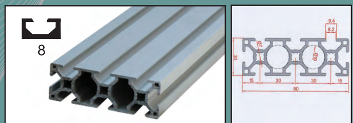
30X90 profile
