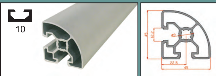
45X45 radius
